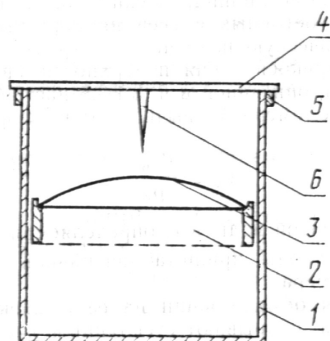
1 - цилиндрический сосуд; 2 - пригружающий пуансон; 3 - петля; 4 - металлическая пластина; 5 - ограничители; 6 - стрелка.
